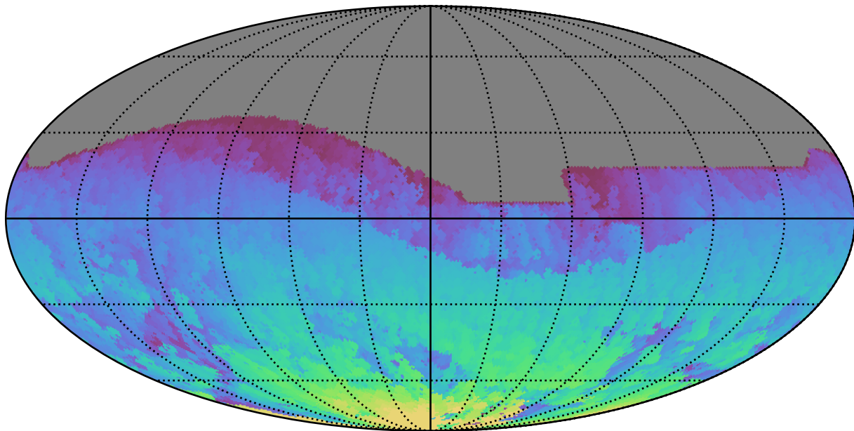
no_magell_roll_v3.4_10yrs All sky z band: Max HA
