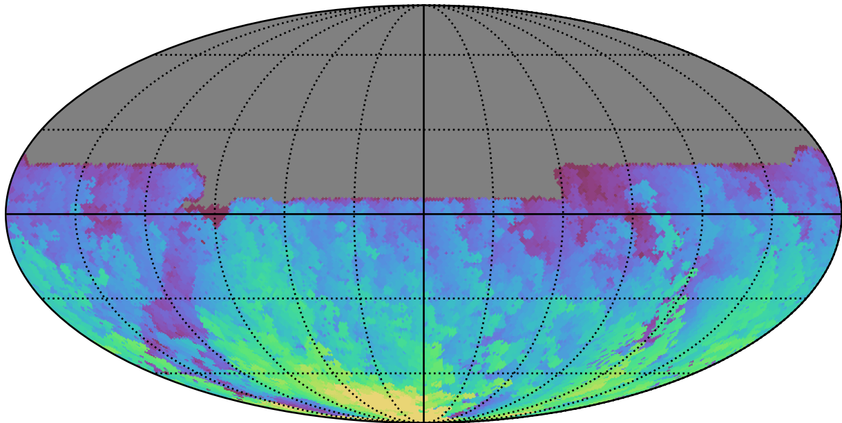
no_magell_roll_v3.4_10yrs All sky u band: Max HA
