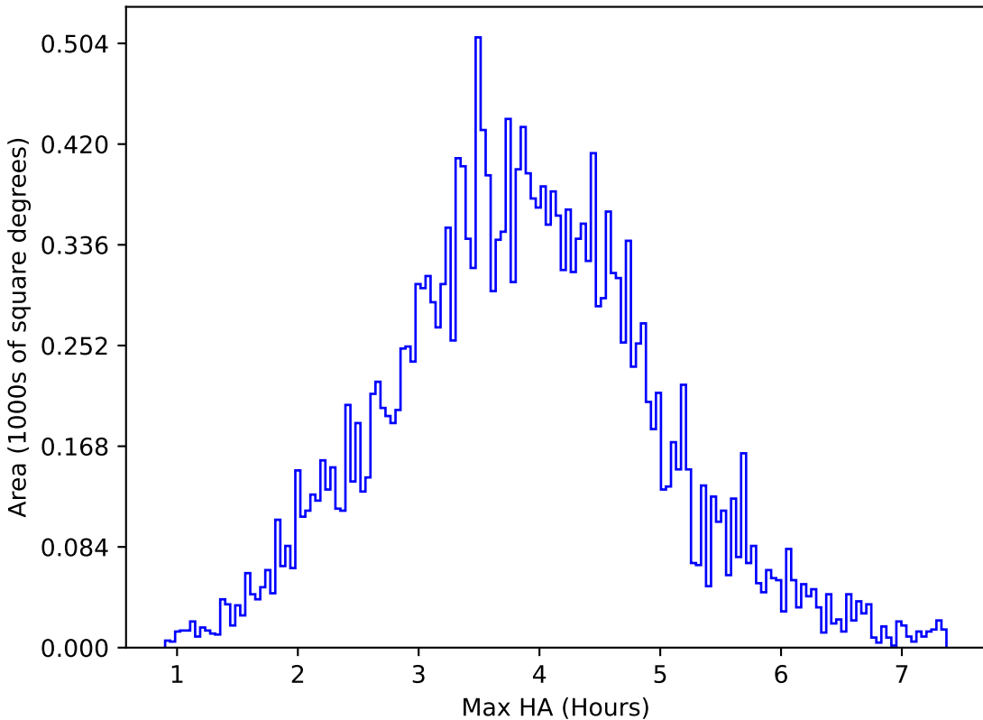
no_magell_roll_v3.4_10yrs All sky u band: Max HA
