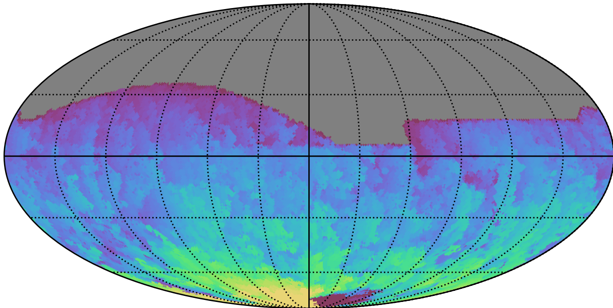
no_magell_roll_v3.4_10yrs All sky r band: Max HA
