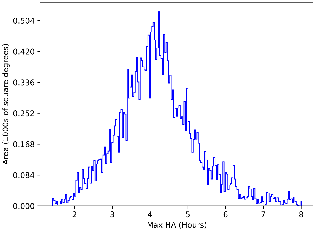
no_magell_roll_v3.4_10yrs All sky r band: Max HA
