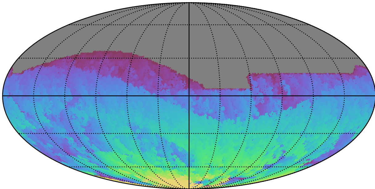
no_magell_roll_v3.4_10yrs All sky i band: Max HA
