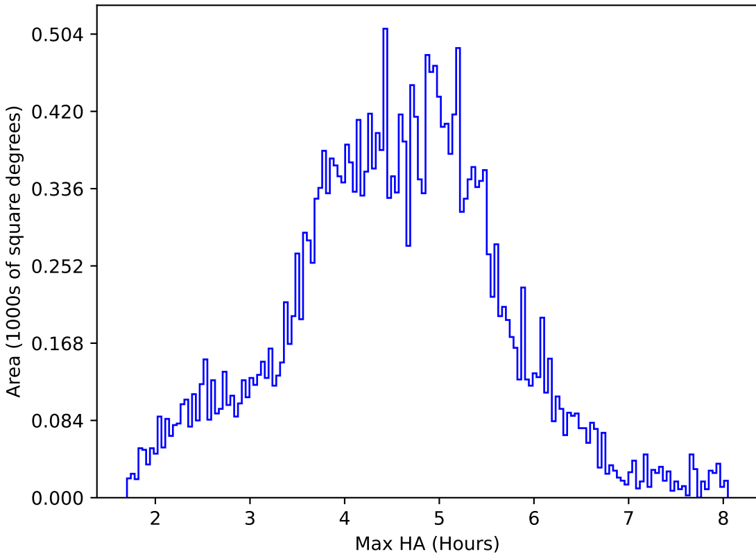
no_magell_roll_v3.4_10yrs All sky i band: Max HA
