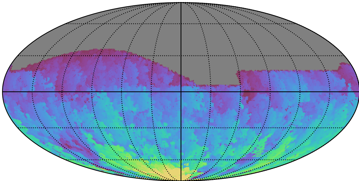
no_magell_roll_v3.4_10yrs All sky g band: Max HA
