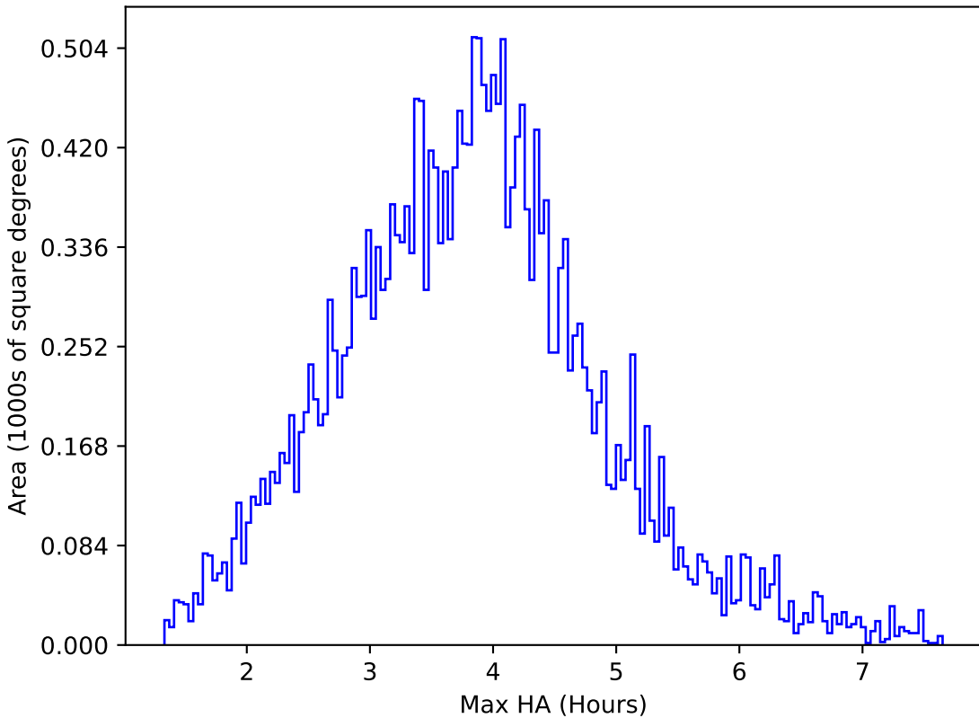
no_magell_roll_v3.4_10yrs All sky g band: Max HA
