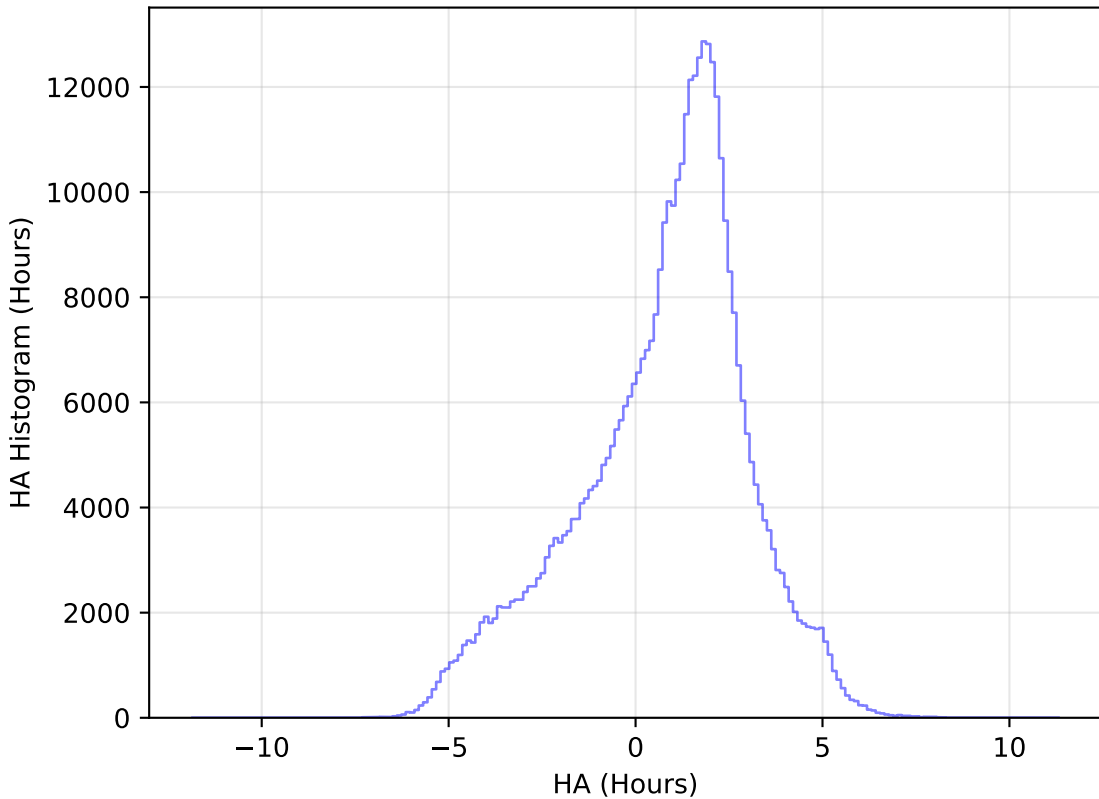
no_magell_roll_v3.4_10yrs WFD z band: HA Histogram
