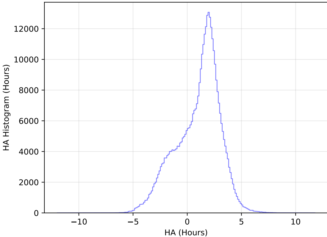
no_magell_roll_v3.4_10yrs WFD y band: HA Histogram
