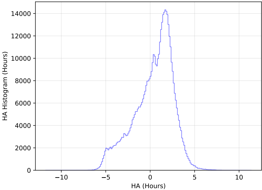
no_magell_roll_v3.4_10yrs WFD r band: HA Histogram
