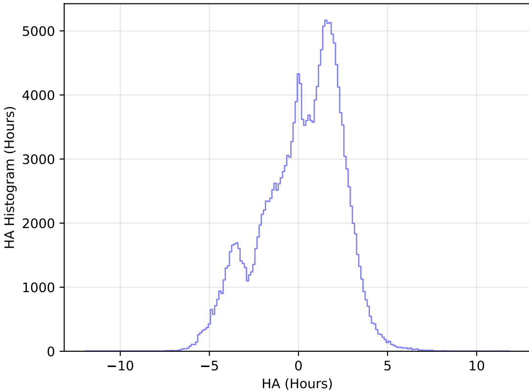
no_magell_roll_v3.4_10yrs WFD g band: HA Histogram
