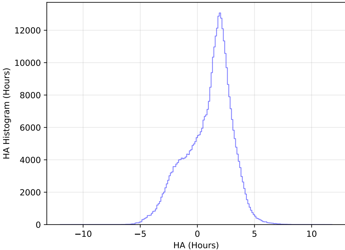
no_magell_roll_v3.4_10yrs All sky y band: HA Histogram
