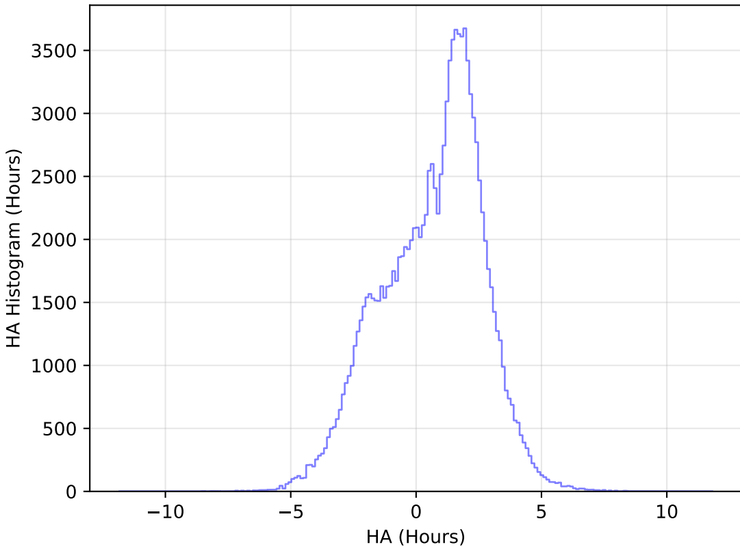
no_magell_roll_v3.4_10yrs All sky u band: HA Histogram
