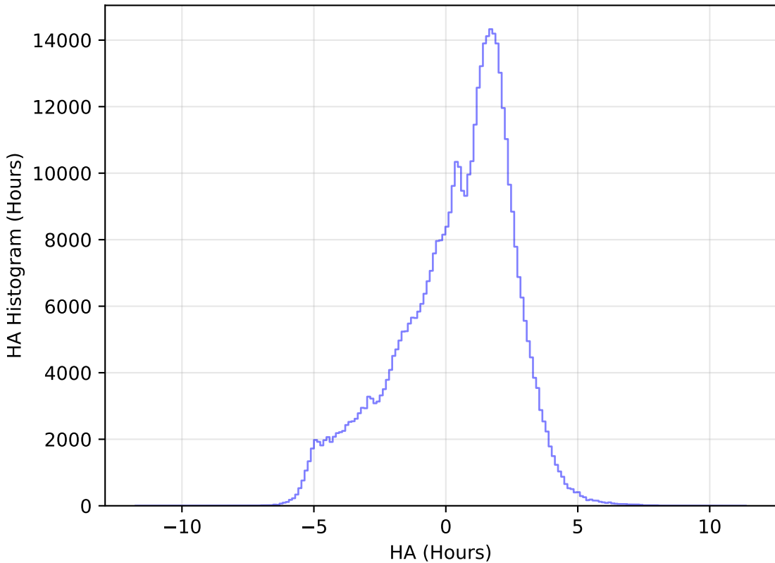
no_magell_roll_v3.4_10yrs All sky r band: HA Histogram
