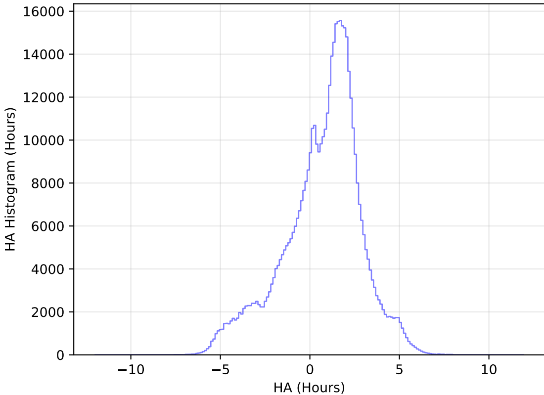
no_magell_roll_v3.4_10yrs All sky i band: HA Histogram
