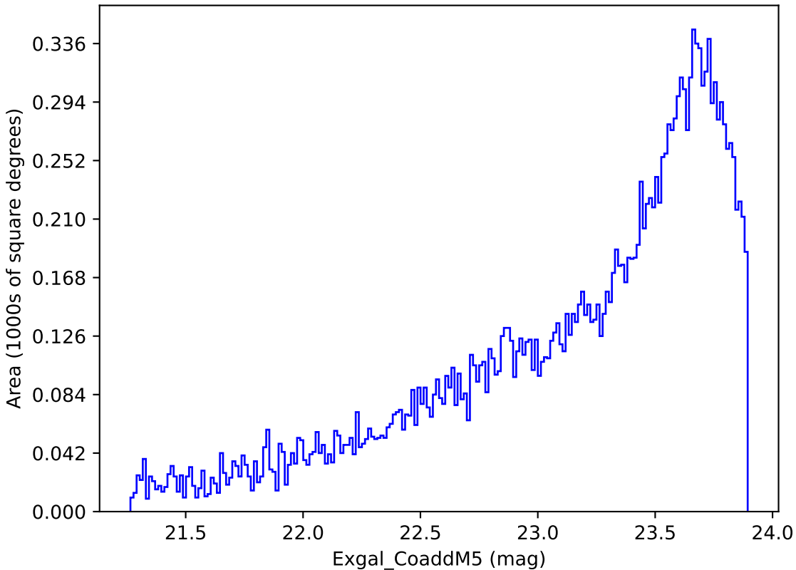
no_magell_roll_v3.4_10yrs Yr 3-4 y band: Exgal_CoaddM5
