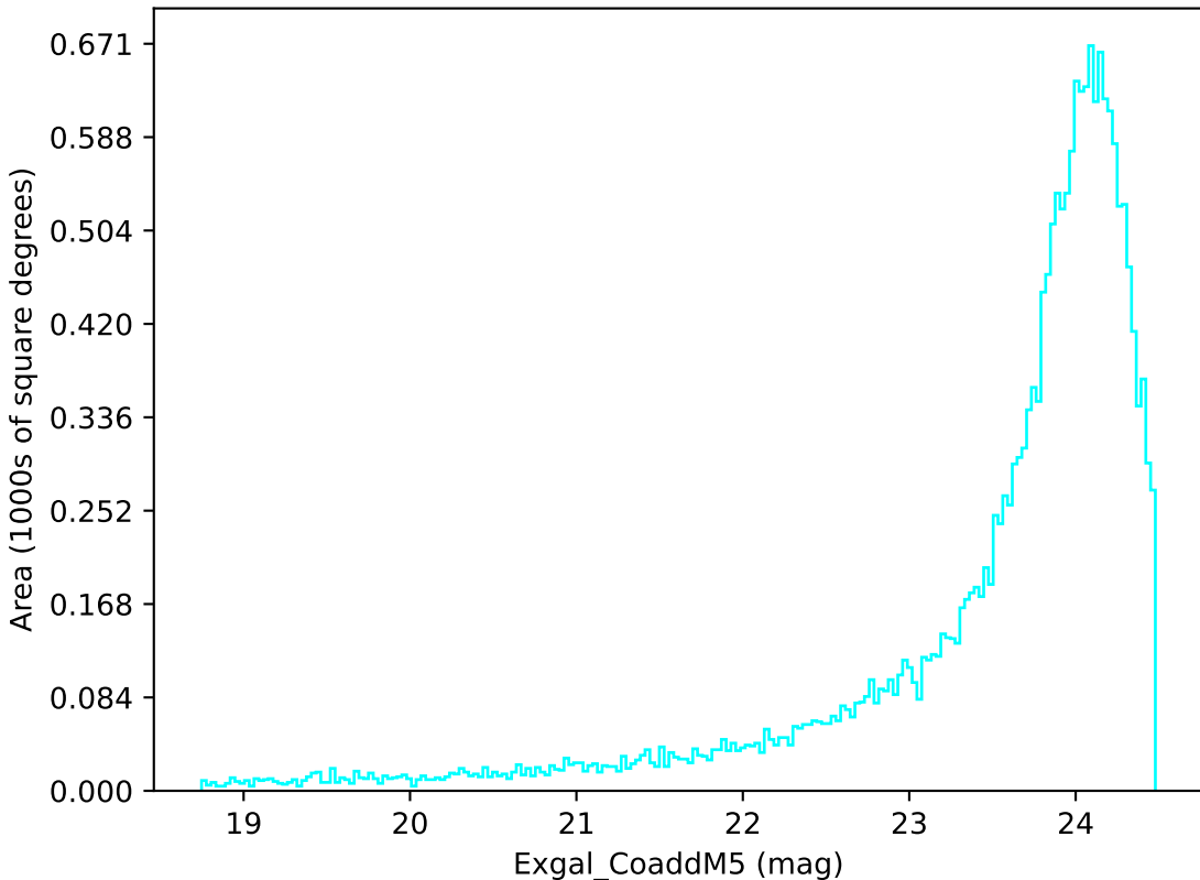
no_magell_roll_v3.4_10yrs Yr 1 u band: Exgal_CoaddM5
