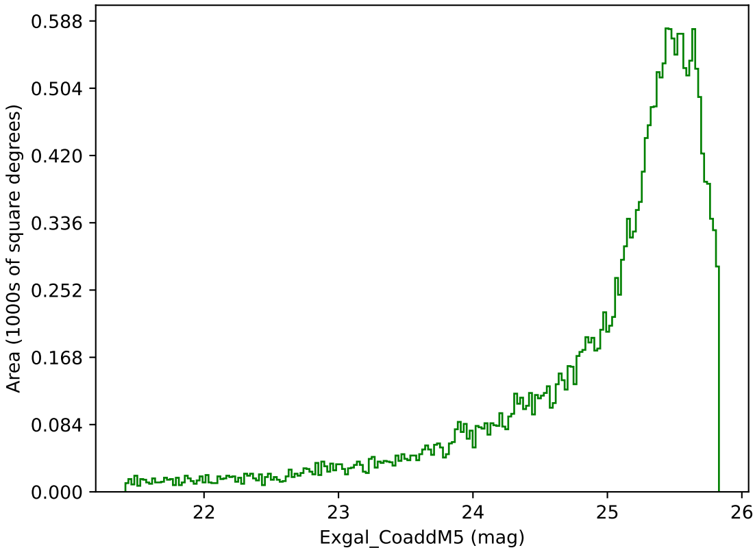
no_magell_roll_v3.4_10yrs Yr 1 g band: Exgal_CoaddM5
