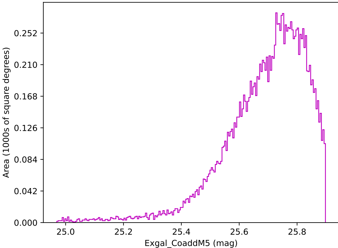
no_magell_roll_v3.4_10yrs WFD z band: Exgal_CoaddM5
