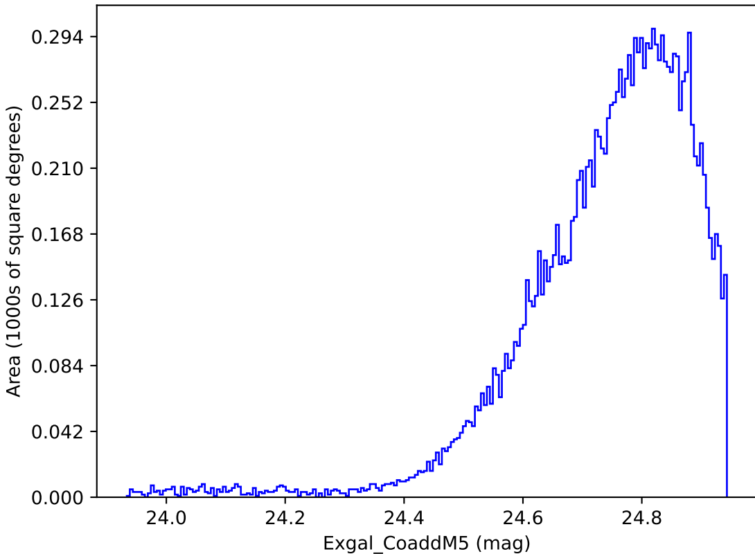
no_magell_roll_v3.4_10yrs WFD y band: Exgal_CoaddM5
