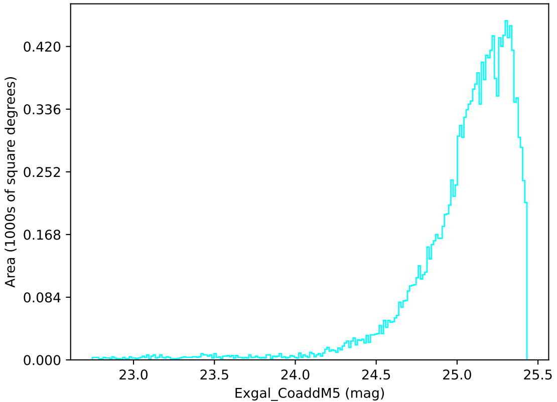
no_magell_roll_v3.4_10yrs WFD u band: Exgal_CoaddM5
