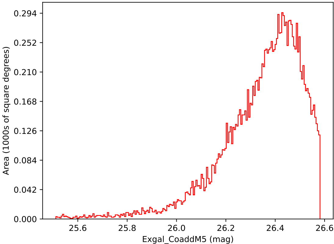
no_magell_roll_v3.4_10yrs WFD i band: Exgal_CoaddM5
