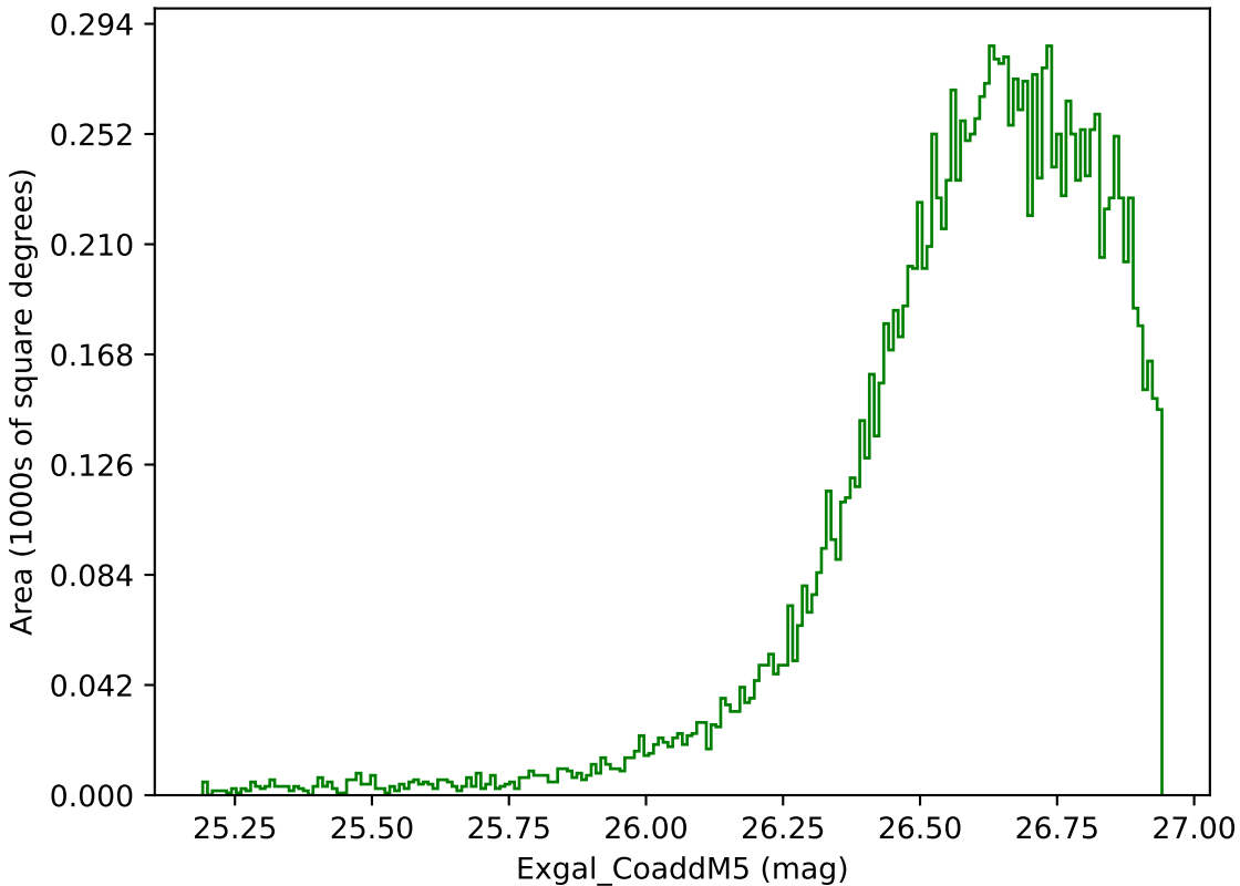
no_magell_roll_v3.4_10yrs WFD g band: Exgal_CoaddM5
