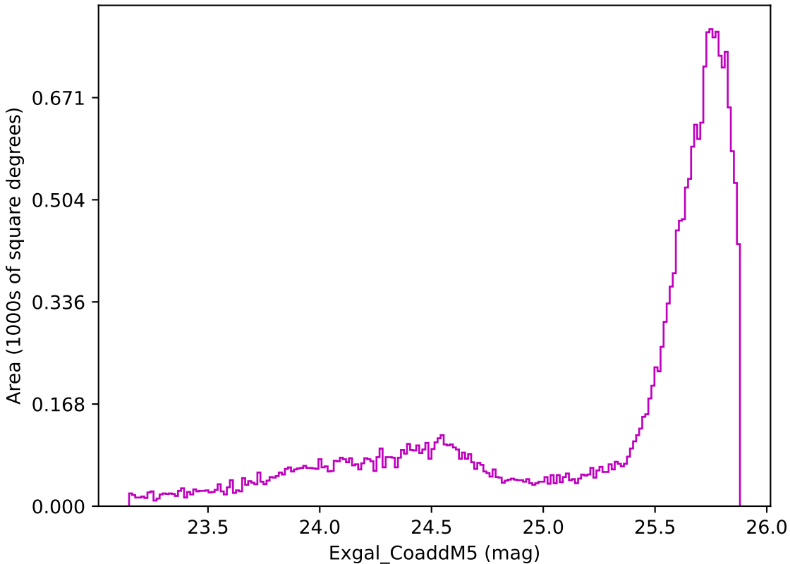
no_magell_roll_v3.4_10yrs All sky z band: Exgal_CoaddM5
