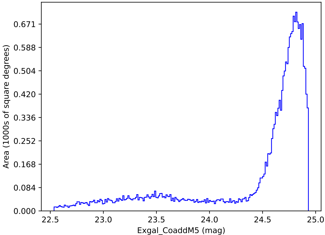
no_magell_roll_v3.4_10yrs All sky y band: Exgal_CoaddM5
