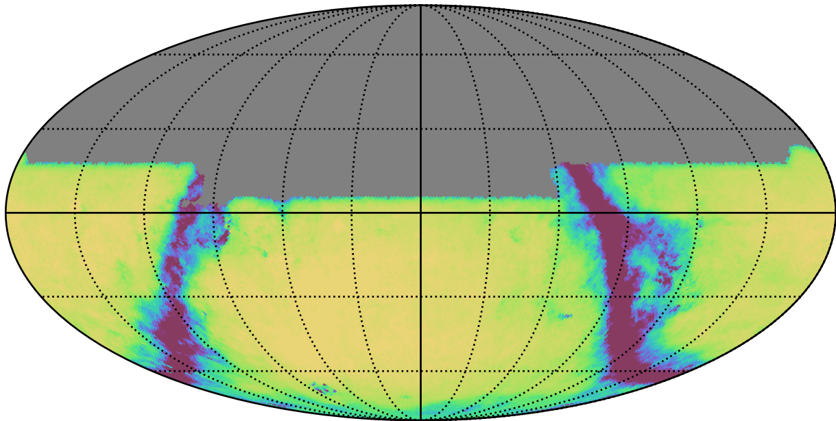
no_magell_roll_v3.4_10yrs All sky u band: Exgal_CoaddM5
