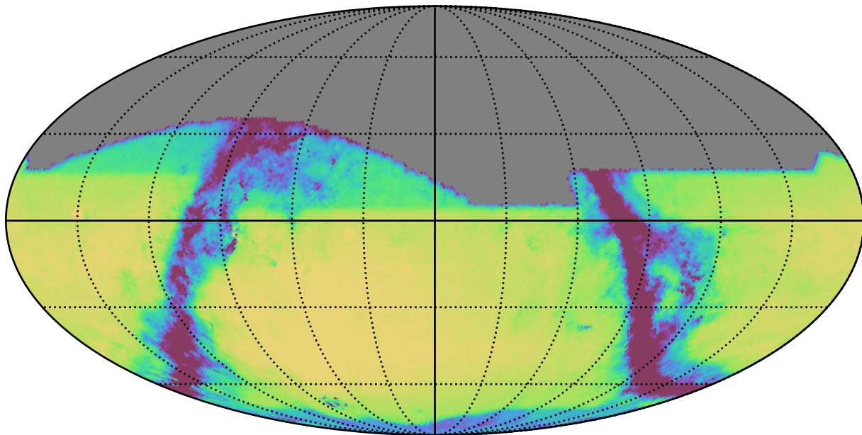
no_magell_roll_v3.4_10yrs All sky r band: Exgal_CoaddM5
