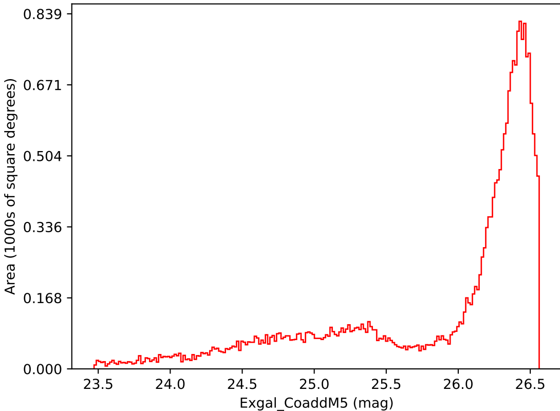
no_magell_roll_v3.4_10yrs All sky i band: Exgal_CoaddM5
