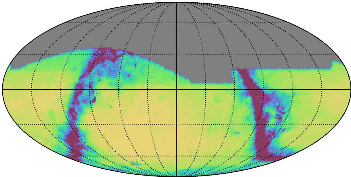
no_magell_roll_v3.4_10yrs All sky g band: Exgal_CoaddM5
