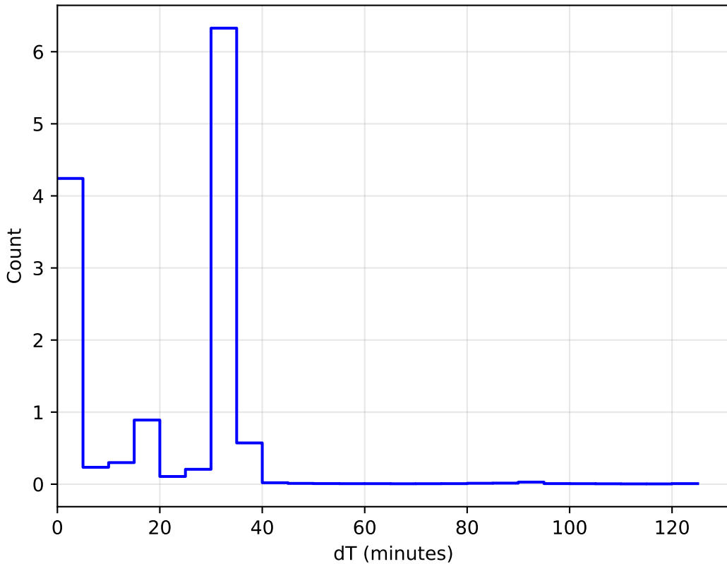
1e6 no_magell_roll_v3.4_10yrs All sky: DeltaT Histogram
