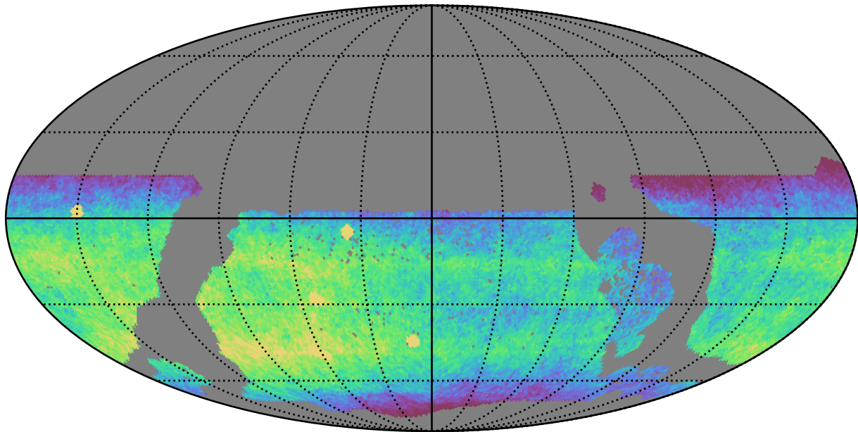
no_magell_roll_v3.4_10yrs WFD z band: CoaddM5
