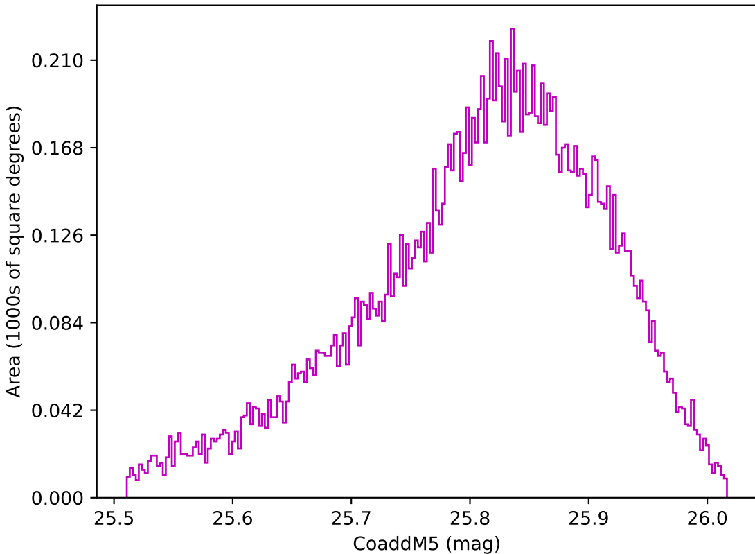
no_magell_roll_v3.4_10yrs WFD z band: CoaddM5
