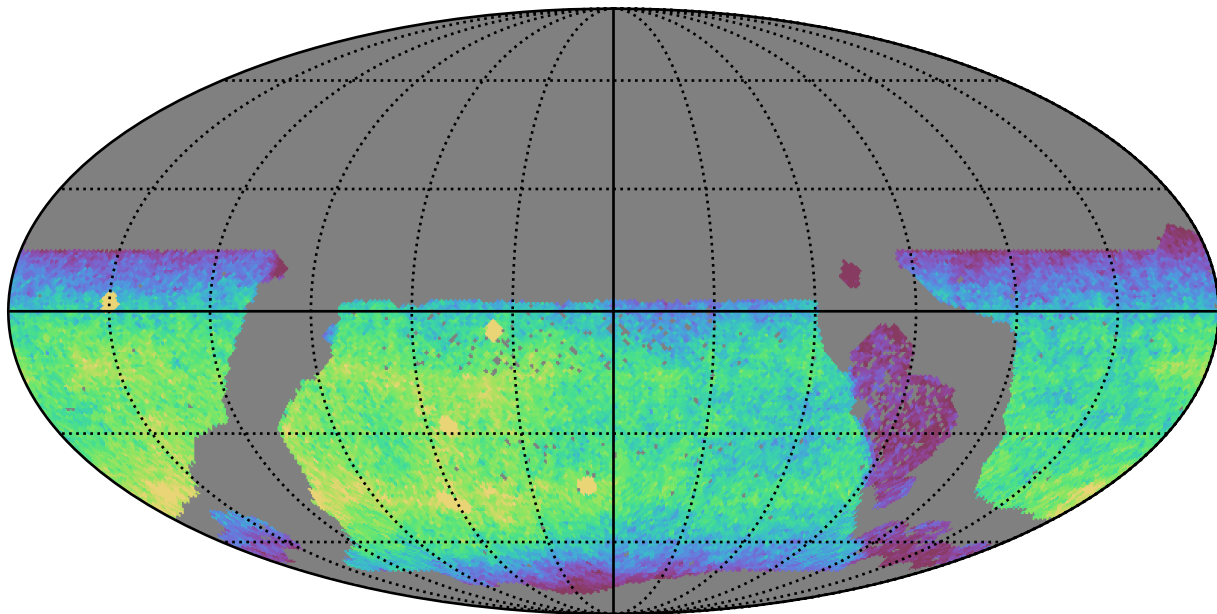
no_magell_roll_v3.4_10yrs WFD y band: CoaddM5
