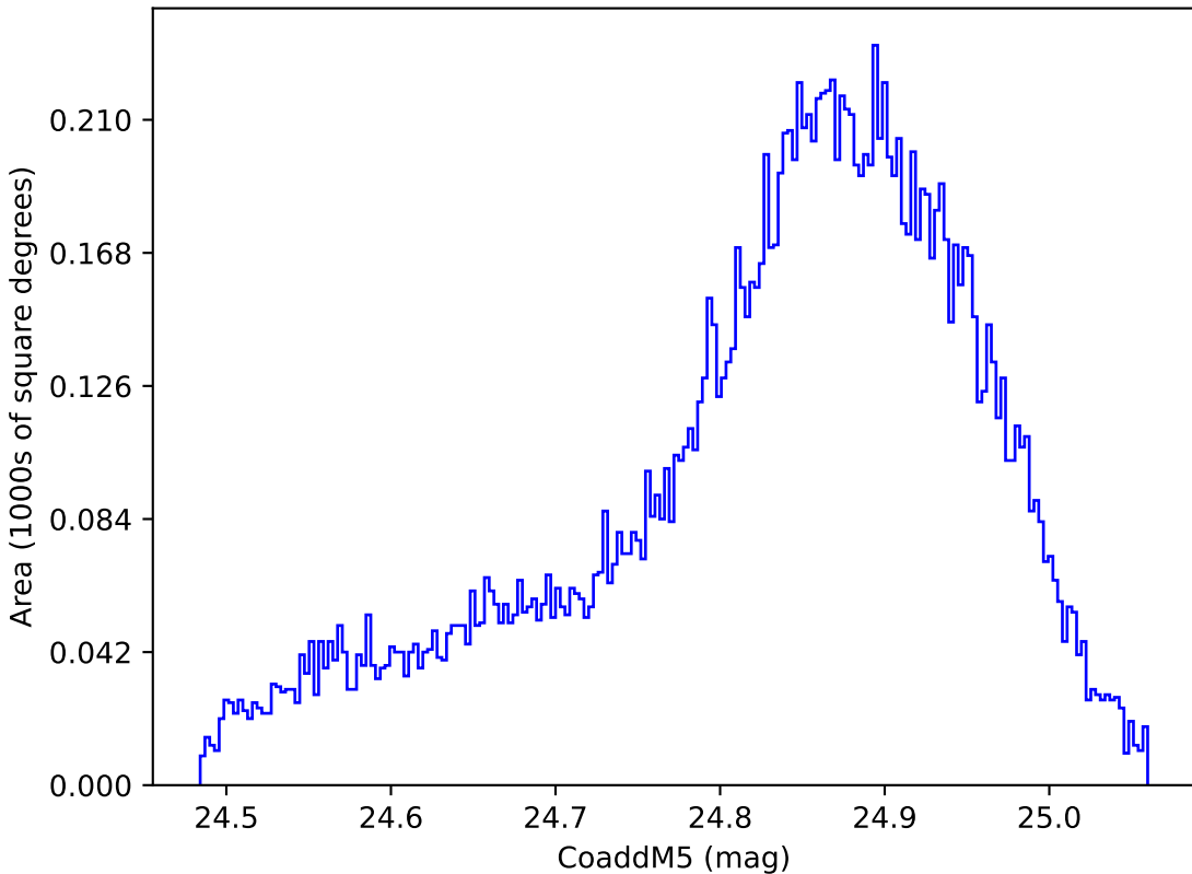
no_magell_roll_v3.4_10yrs WFD y band: CoaddM5
