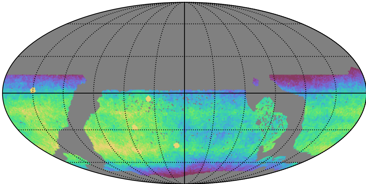
no_magell_roll_v3.4_10yrs WFD i band: CoaddM5
