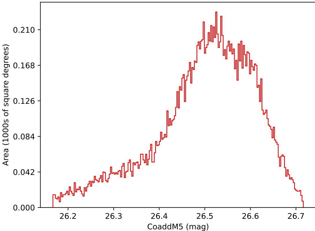
no_magell_roll_v3.4_10yrs WFD i band: CoaddM5
