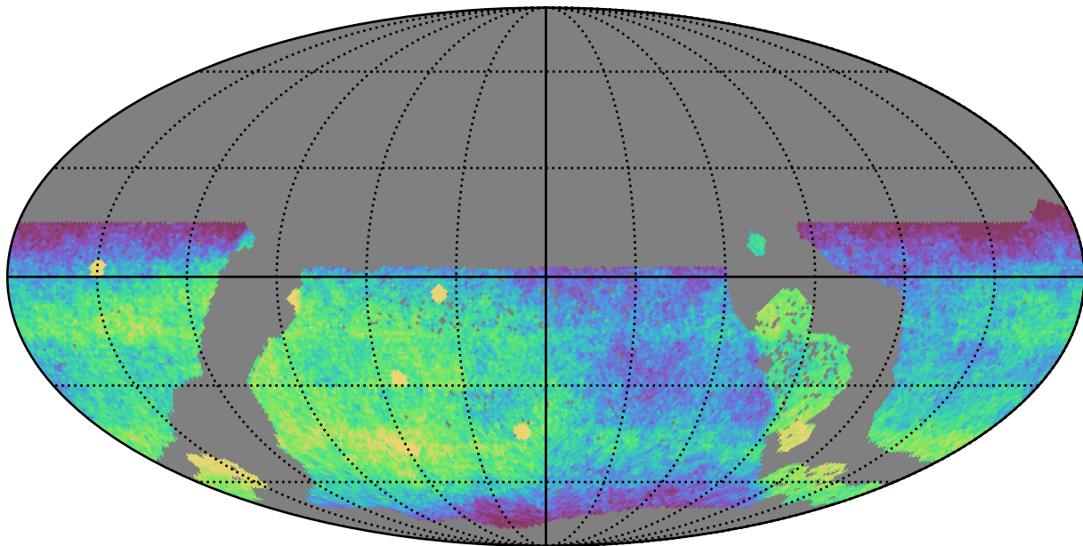
no_magell_roll_v3.4_10yrs WFD g band: CoaddM5
