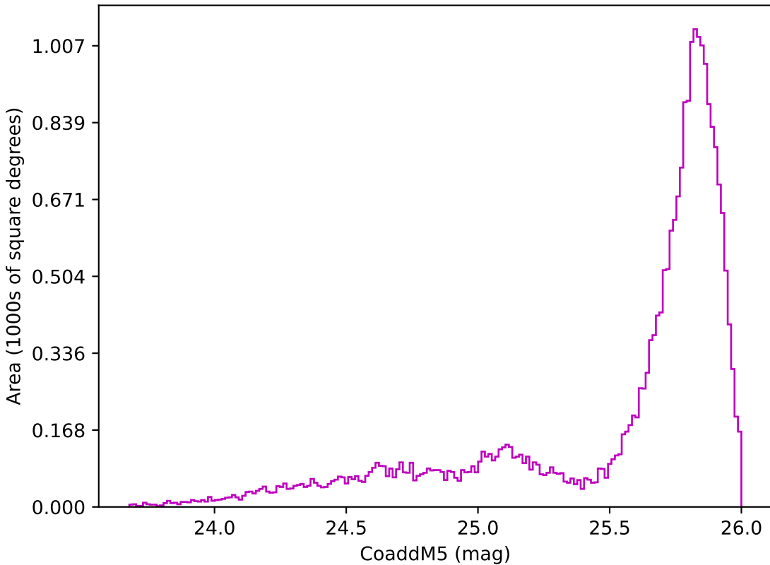
no_magell_roll_v3.4_10yrs All sky z band: CoaddM5
