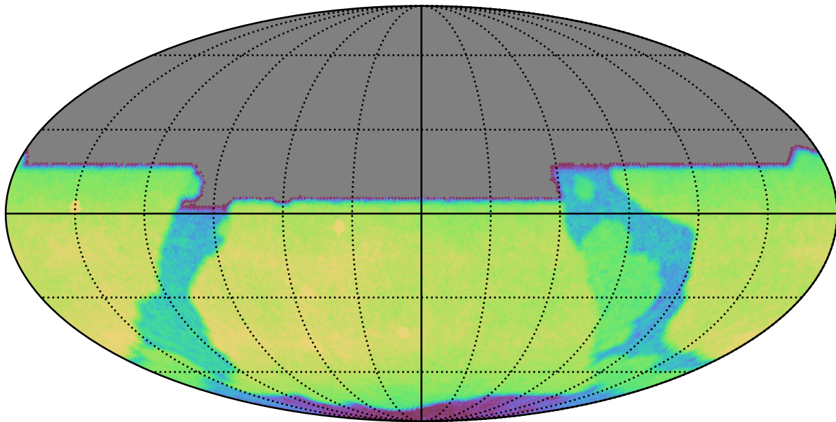
no_magell_roll_v3.4_10yrs All sky y band: CoaddM5
