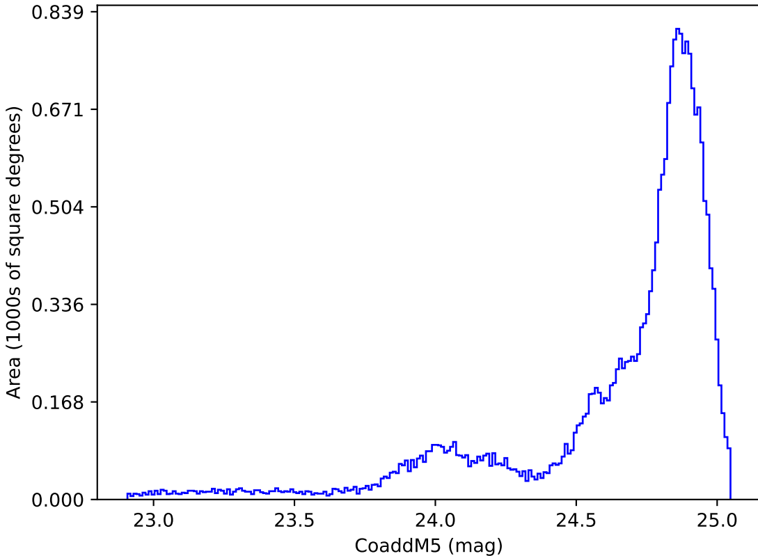
no_magell_roll_v3.4_10yrs All sky y band: CoaddM5
