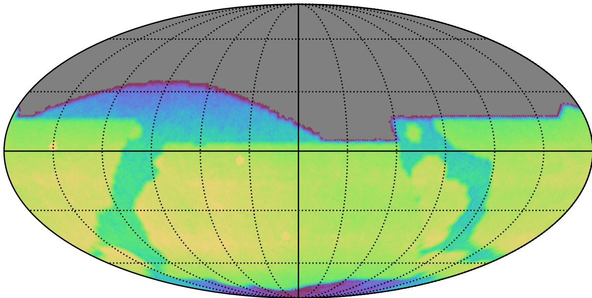
no_magell_roll_v3.4_10yrs All sky r band: CoaddM5
