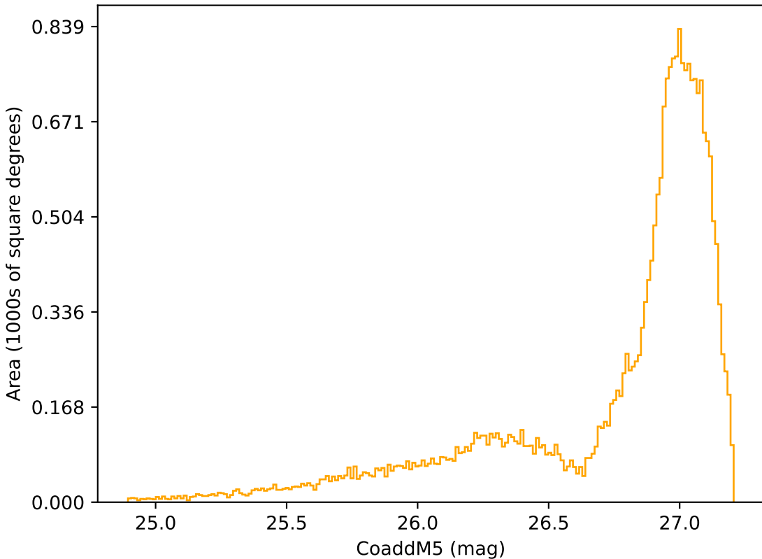
no_magell_roll_v3.4_10yrs All sky r band: CoaddM5
