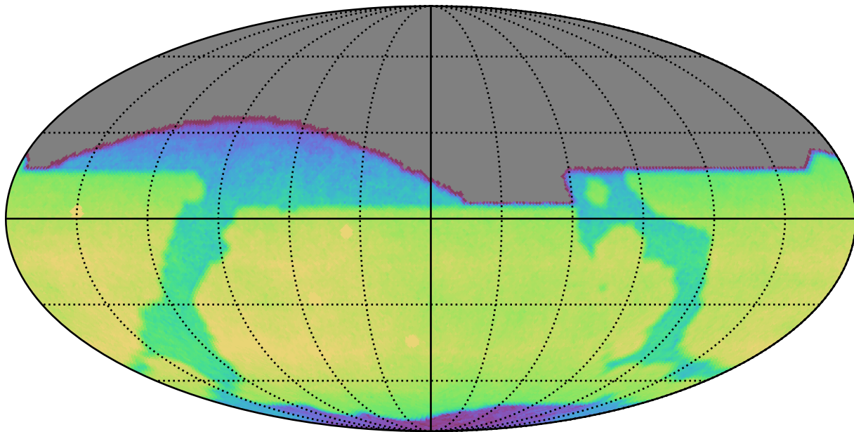
no_magell_roll_v3.4_10yrs All sky i band: CoaddM5
