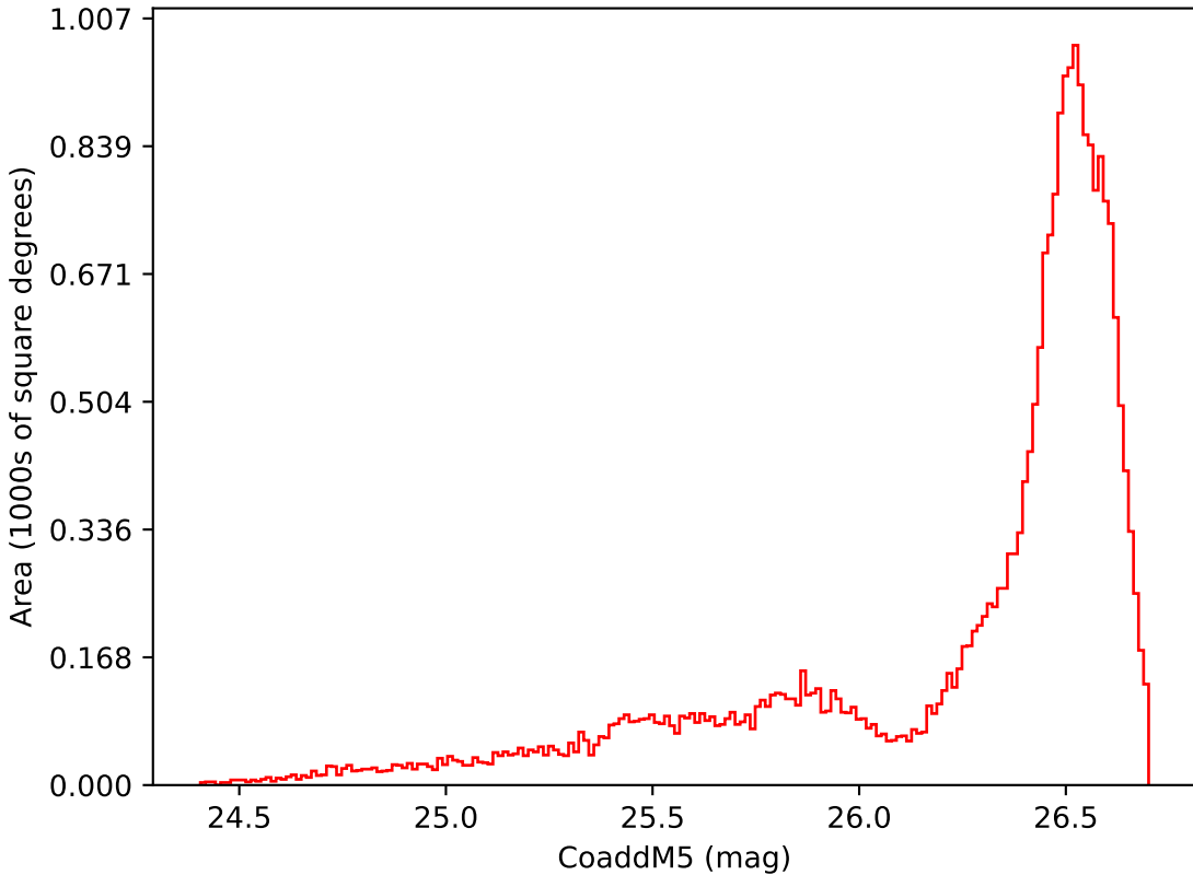
no_magell_roll_v3.4_10yrs All sky i band: CoaddM5
