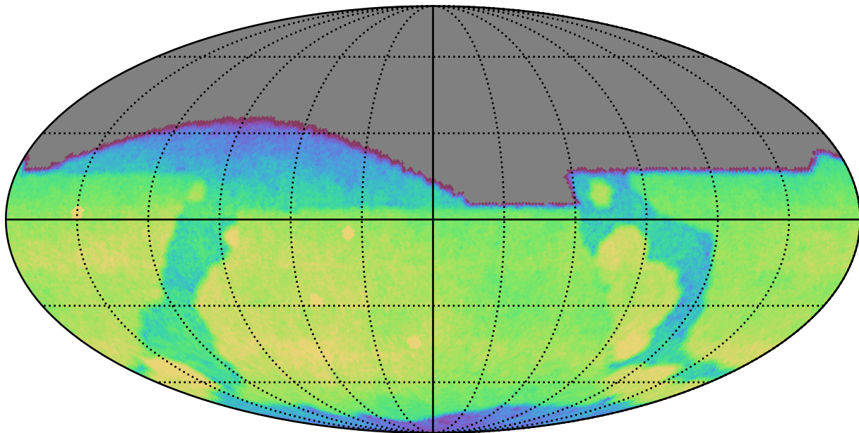
no_magell_roll_v3.4_10yrs All sky g band: CoaddM5
