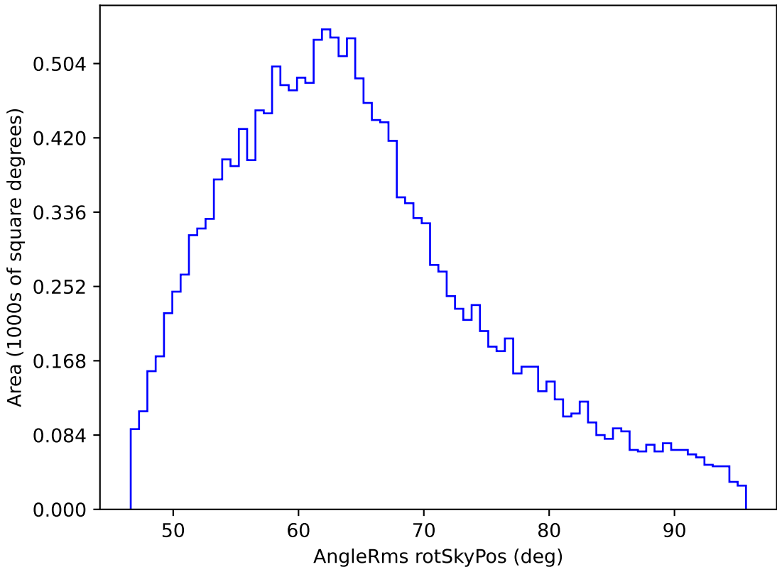
no_magell_roll_v3.4_10yrs WFD z band: AngleRms rotSkyPos
