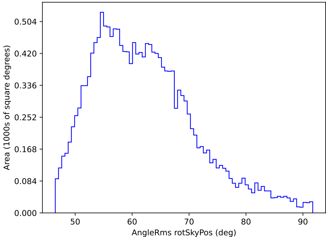
no_magell_roll_v3.4_10yrs WFD y band: AngleRms rotSkyPos
