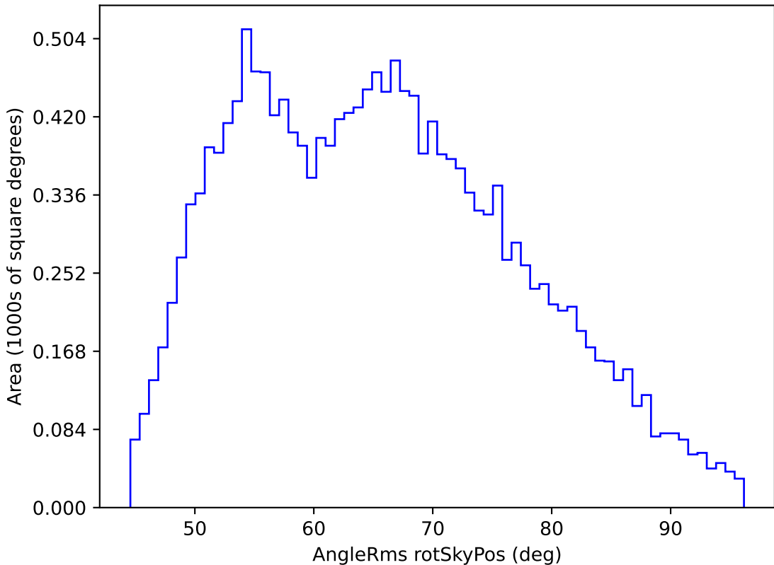
no_magell_roll_v3.4_10yrs WFD u band: AngleRms rotSkyPos
